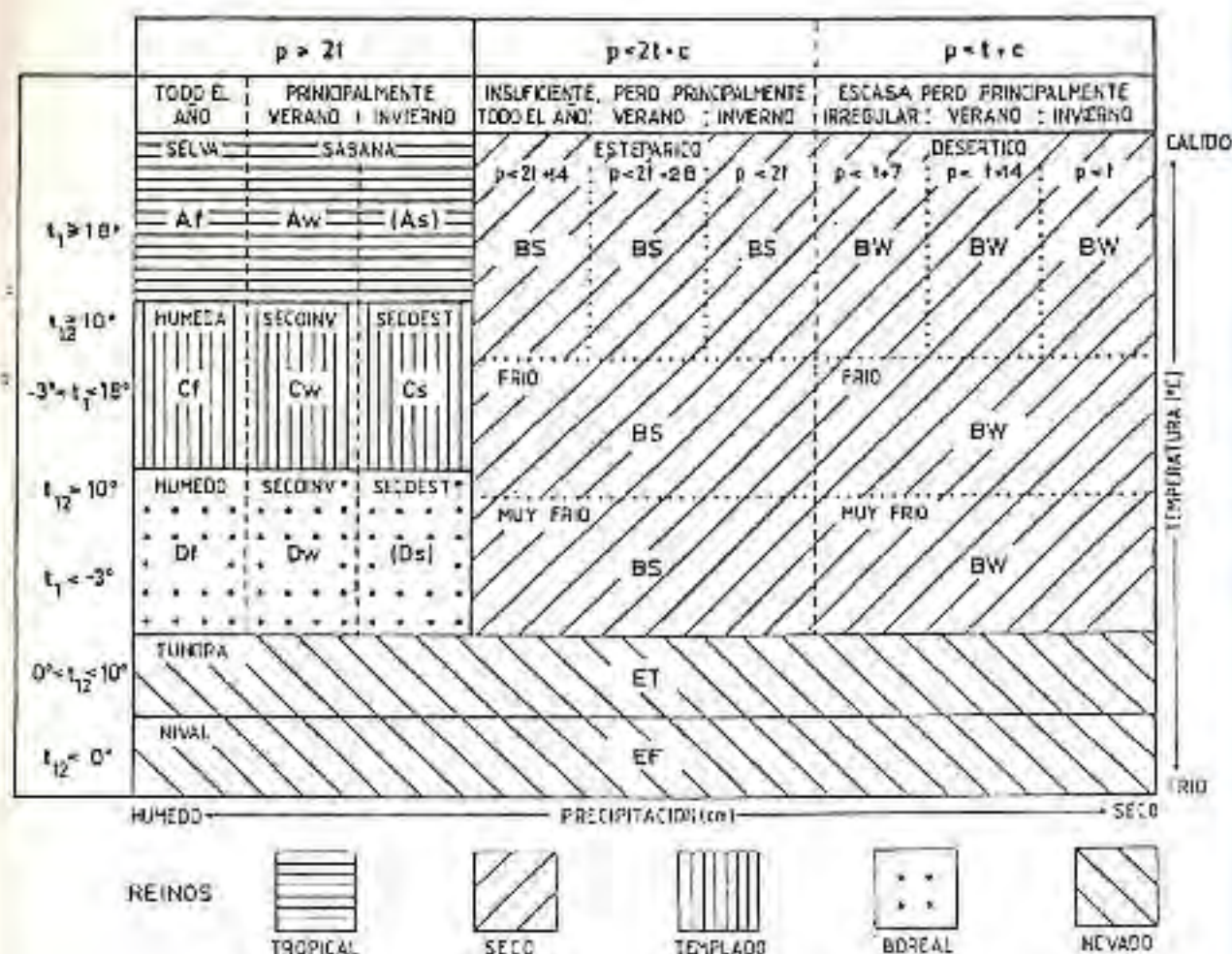
Figura 5. Esquema de las relaciones entre temperatura y humedad que caracterizan a los Reinos y Dominios de pastizales. (Basado en Höppen 1948 y Peña y Schneider 1982, modificada por los autores).
